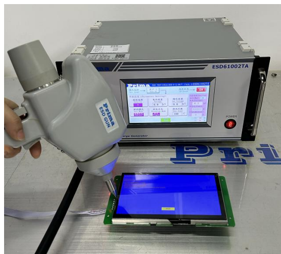
图 5-2 ESD 测试图
