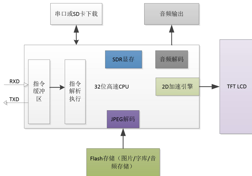
图 9-1 HMI 硬件结构参考图
