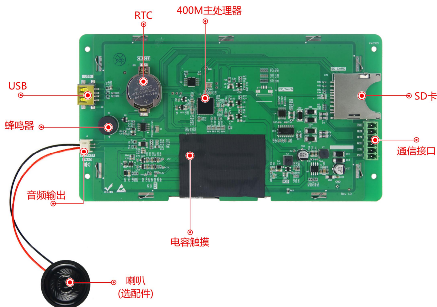
图 1-2 硬件配置图
