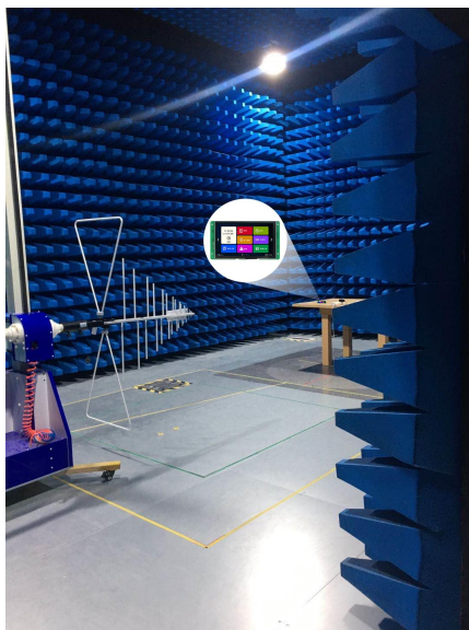
图 5-5 辐射测试图
